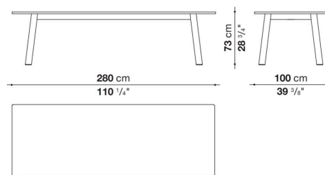
TBU280M
