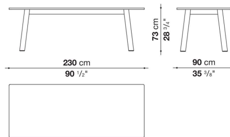
TBU230M
