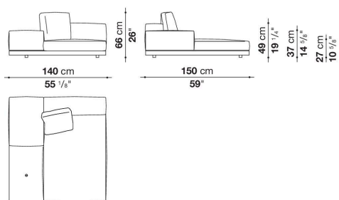
DBL150LS_2
