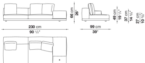
DBL230TD_3
