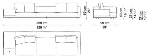
DB329S_2
