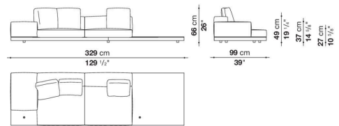
DBL329AD_4
