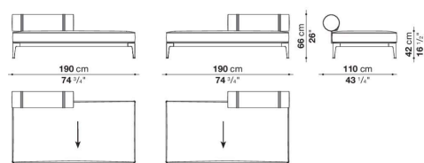
RBR190PA
