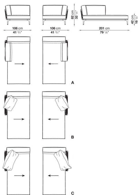
RB201LB_1
