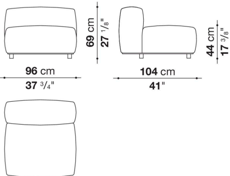
DU96C
