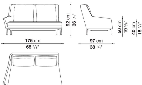
ED176TAS_V
