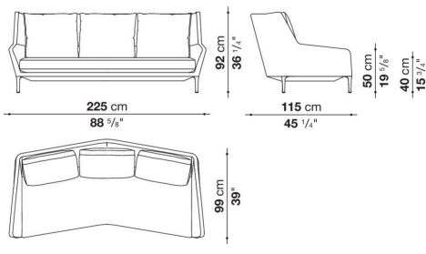
ED225_V
