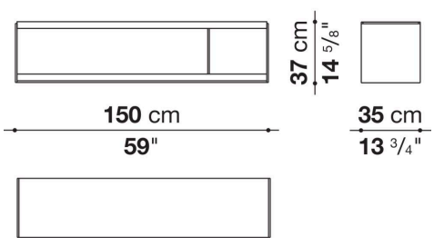
TSF150A
