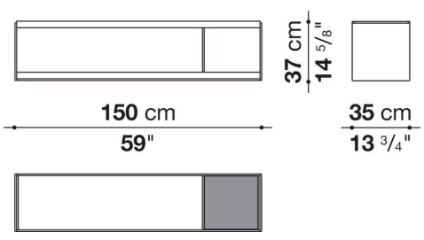
TSF150AV
